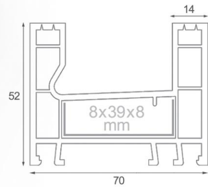
Code 7101 MW Series (Sliding) پروفیل فریم دو ریل کشویی Sliding frame profile
