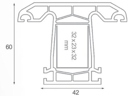
Series (4 Chamber) پروفیل میانی ثابت Mullion profile 60mm
