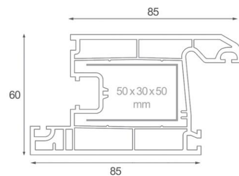
Series (3 Chamber) پروفیل لنگه داخل بازشوی درب In Door Sash profile 60mm
