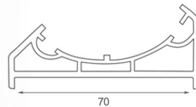
Code 5753 MW Series پروفیل آداپتور لوله Pipe Adaptor profile 70mm
