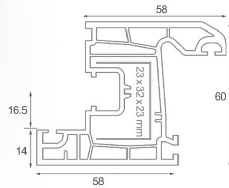
Series (4 Chamber) پروفیل لنگه پنجره Sash profile 60mm
