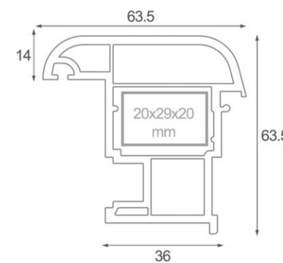
Series (4 Chamber) پروفیل میانی متحرک False Mullion profile 60mm
