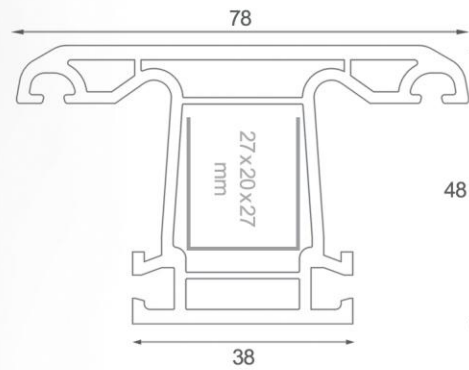
8004 (NW/GW) Series (Sliding) پروفیل میانی کشویی Sliding Mullion profile
