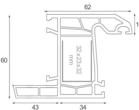
Series (4 Chamber) پروفیل قاب باز سازی Renovation Frame profile 60mm
