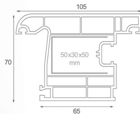
Series (4 Chamber) پروفیل لنگه بیرون بازشوی درب Out Door Sash profile 70mm
