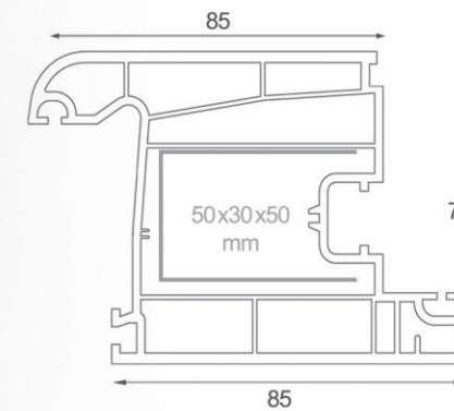
Code 7007 NW/GW Series (4 Chamber) پروفیل لنگه داخل بازشوی درب In Door Sash profile 70mm
