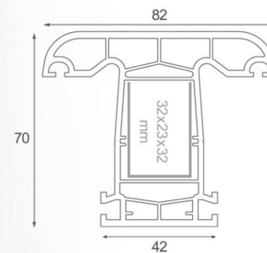
Series (5 Chamber) پروفیل میانی ثابت Mullion profile 70mm
