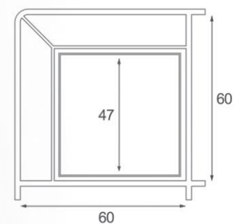
Code 5654 MW Series پروفیل قوطی Box profile 60mm
