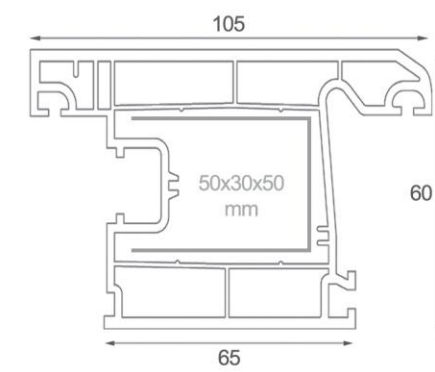
Series (3 Chamber) پروفیل لنگه بیرون بازشوی درب Out Door Sash profile 60mm
