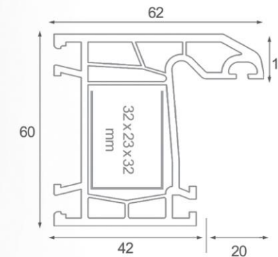
Series (4 Chamber) پروفیل فریم پنجره Normal Frame profile 60mm
