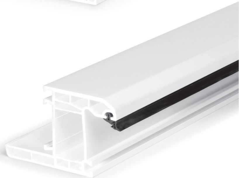
Series (4 Chamber) پروفیل قاب باز سازی Renovation Frame profile 60mm
