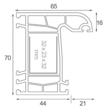
Code 7001 (NW/GW) Series (5 Chamber) پروفیل فریم پنجره Frame profile 70mm
