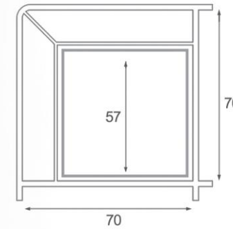
Code 5754 MW Series پروفیل قوطی Box profile 70mm
