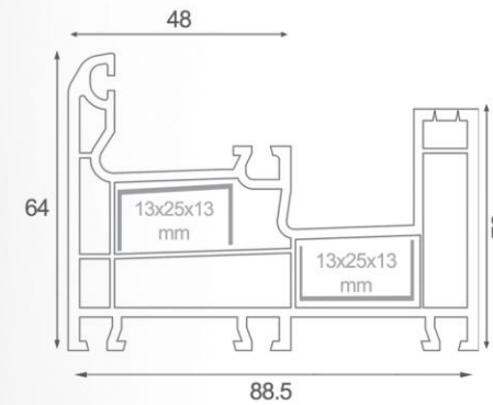
8001 (NW/GW) Series (Sliding) پروفیل فریم تک ریل کشویی Mono Rail Sliding Frame profile
