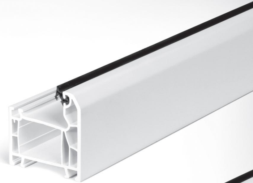
Series (4 Chamber) پروفیل فریم پنجره Normal Frame profile 60mm
