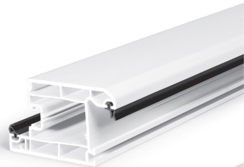
Series (3 Chamber) پروفیل لنگه داخل بازشوی درب In Door Sash profile 60mm
