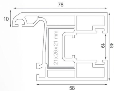
7103 (NW/GW) Series (Sliding) پروفیل لنگه پنجره کشویی Sliding Sash profile
