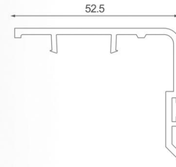
7112 MW Series (Sliding) پروفیل آداپتور لنگه کشویی Sliding Sash Adaptor profile
