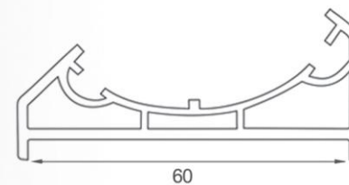
Code 5653 MW Series پروفیل آداپتور لوله Pipe Adaptor profile 60mm
