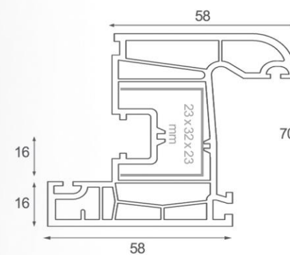
Series (5 Chamber) پروفیل لنگه پنجره Sash profile 70mm
