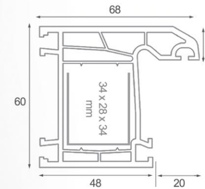
Series (4 Chamber) پروفیل فریم پهن Super Frame profile 60mm
