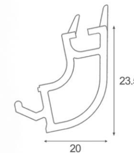
Code 7009 NW/GW Series زهوار شیشه دو جداره Double Glass Glazing bead 70mm
